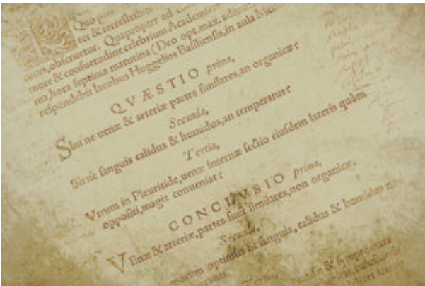
Latein
